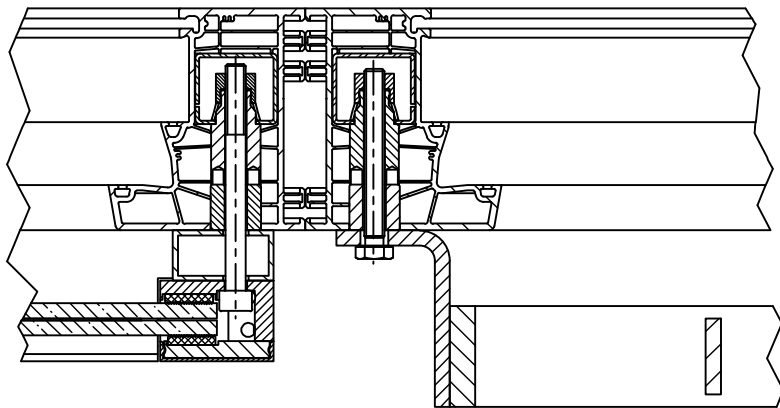
Schnitt A-A
