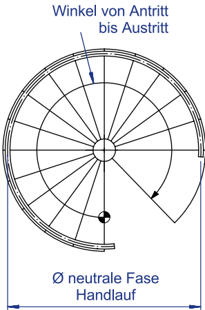
Beispiel Rechtstreppe
