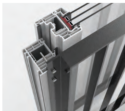
SIMPLUM STAHL IN DER BEFESTIGUNGSVARIANTE EASY AUF EINEM KUNSTSTOFFFENSTER.
