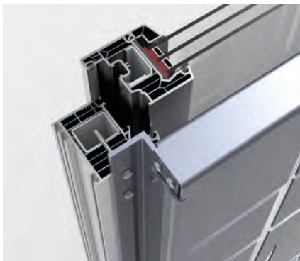
TEMPLATE IN DER BEFESTIGUNG EASY AUF KUNSTSTOFFFENSTER.
