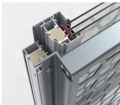
BEFESTIGUNGSVARIANTE CLASSIC MIT PROFILDÜBEL ANCORA.
